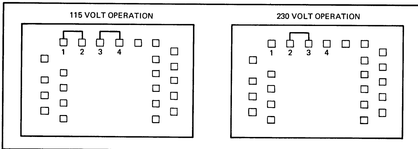
Figure 4-4. 115/230 VOLT CONVERSION
